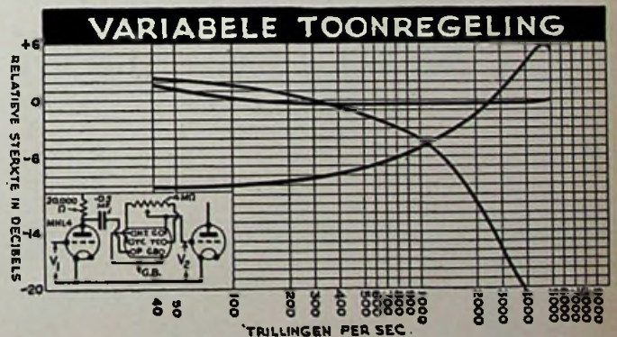
Type 3.5/1. Speciaal ontworpen voor compensatie van hoge toonverlies in selectieve ontvangers en tooncontrole in radio-gramfoon versterkers.
